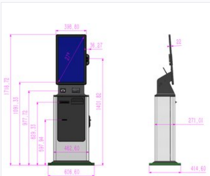
Габариты CRT202 — вид спереди и сбоку
